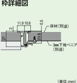
枠詳細図
